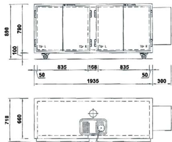
Abmessungen Cocktail Tresen
