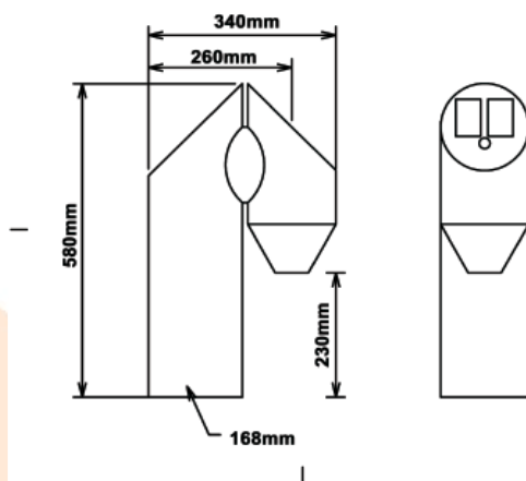
Abmessungen Cocktail Jukebox
